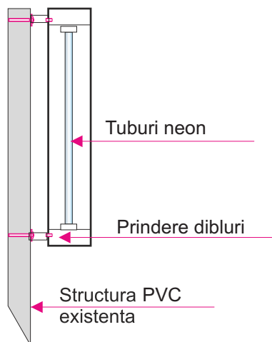
Detaliu fixare caseta pe locatie
