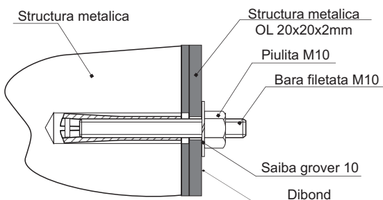
Detaliu fixare caseta pe locatie
